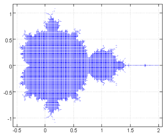
図 5 mandelbrot
