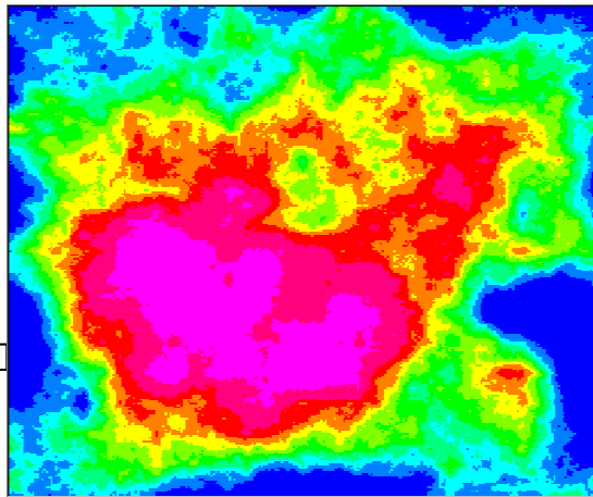
図2 plasma
